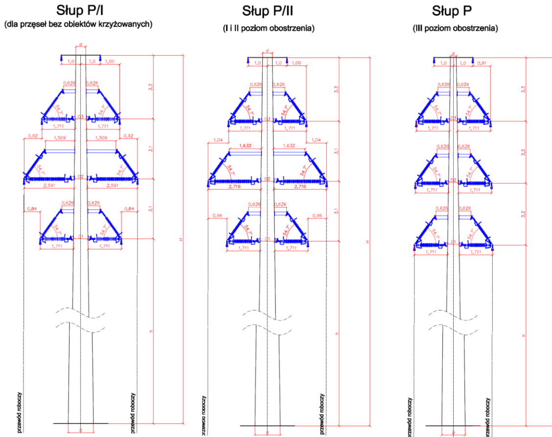
Rys.2. Sylwetki słupów przelotowych linii dwutorowej 110kV dla różnych stopni obciążenia.
